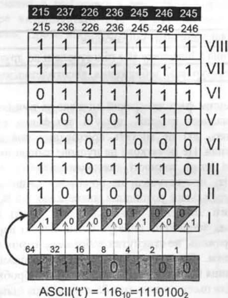
Рис. 1. Ілюстрація принципу стеганографічного приховування інформації у зображеннях
