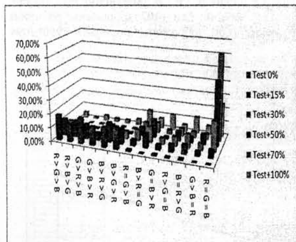
Рис. 5. Залежність нерівностей ПВС від об'єму заповнення НЗБ рівня
