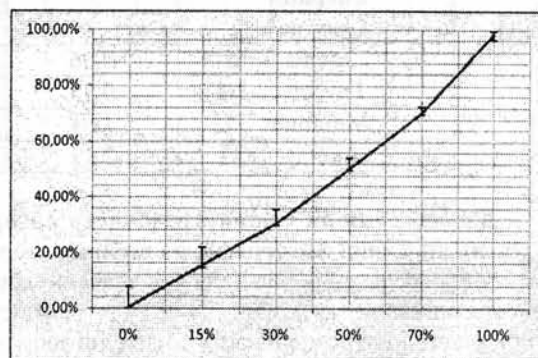
Рис. 4. Залежність ПВС за RS-стегоаналізом від додавання стегобіт у НЗБ
