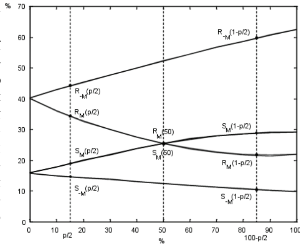
RS -діаграма
